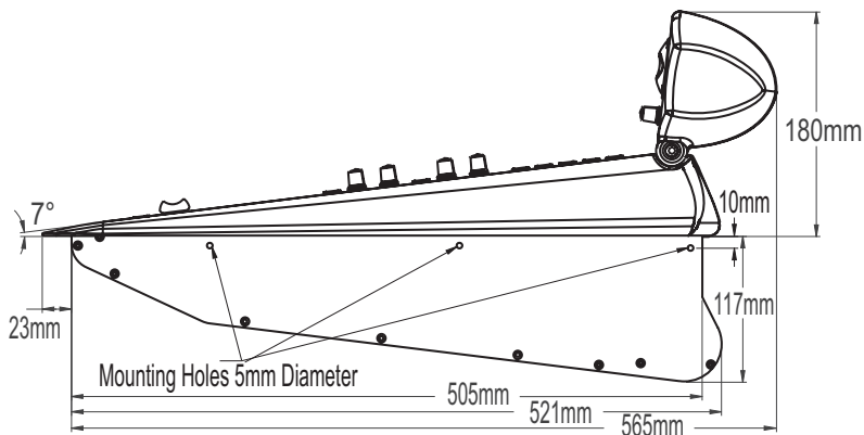
Fig 2-1 : Mixer Profile.
